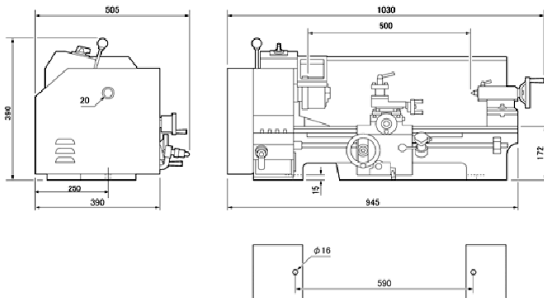
外観2面寸法図
