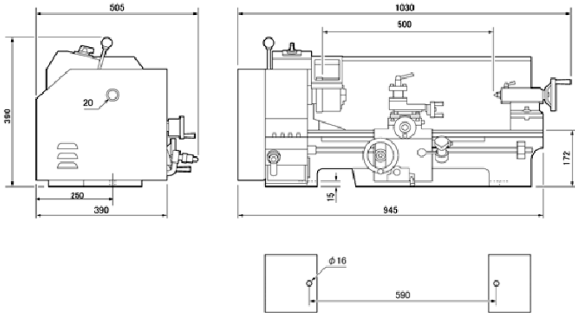
外觀2面寸法図
