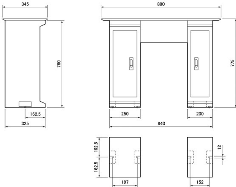
外觀2面寸法図
