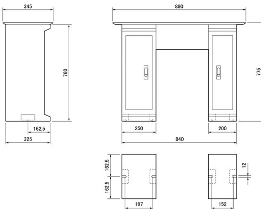
外観2面寸法図
