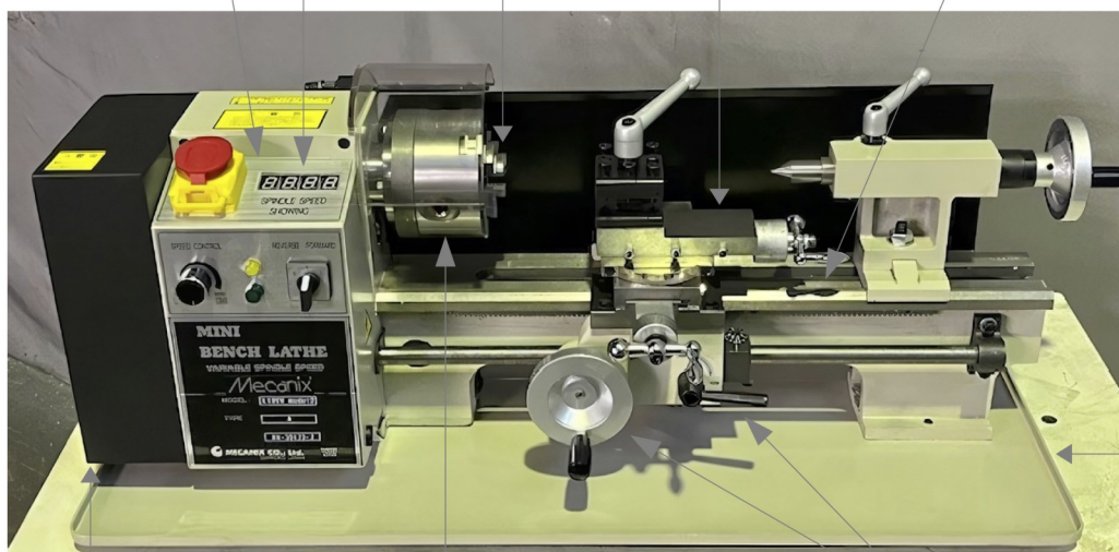
自動送り/ねじ切り装置(左ねじも可)
