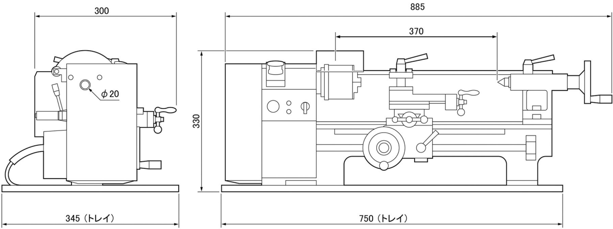
外観2面寸法図
